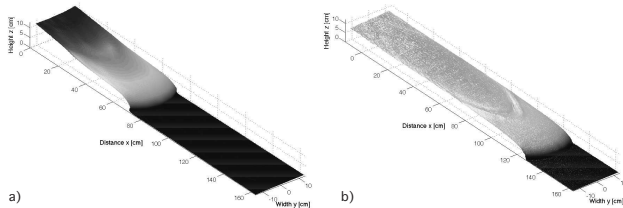
Fig. 21 Free surface at: a) t_1 = 1.0 s, b) t_1 = 52.0 s.
