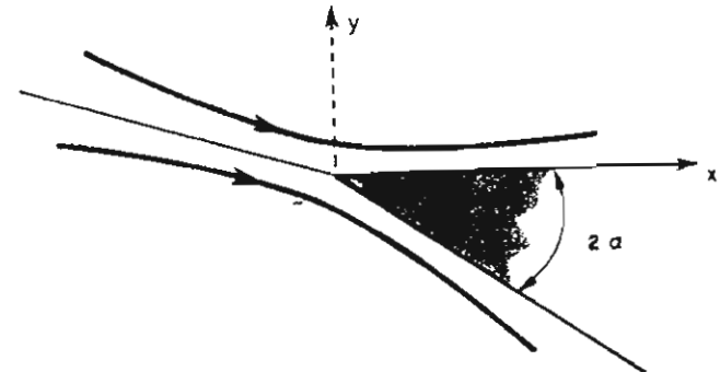
Figure 12 Écoulement autour d'un angle
