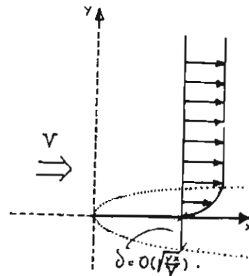
Figure 2 Freinage par une plaque plane
