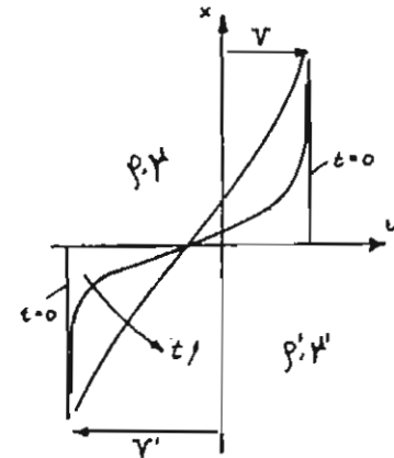
Figure 3 Diffusion d'une surface de contact
